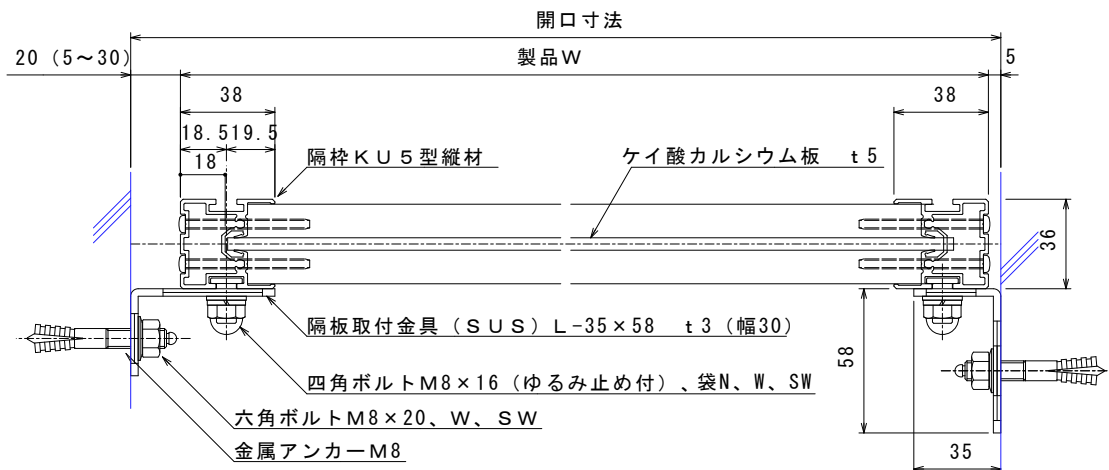
【 横断面詳細図 】
