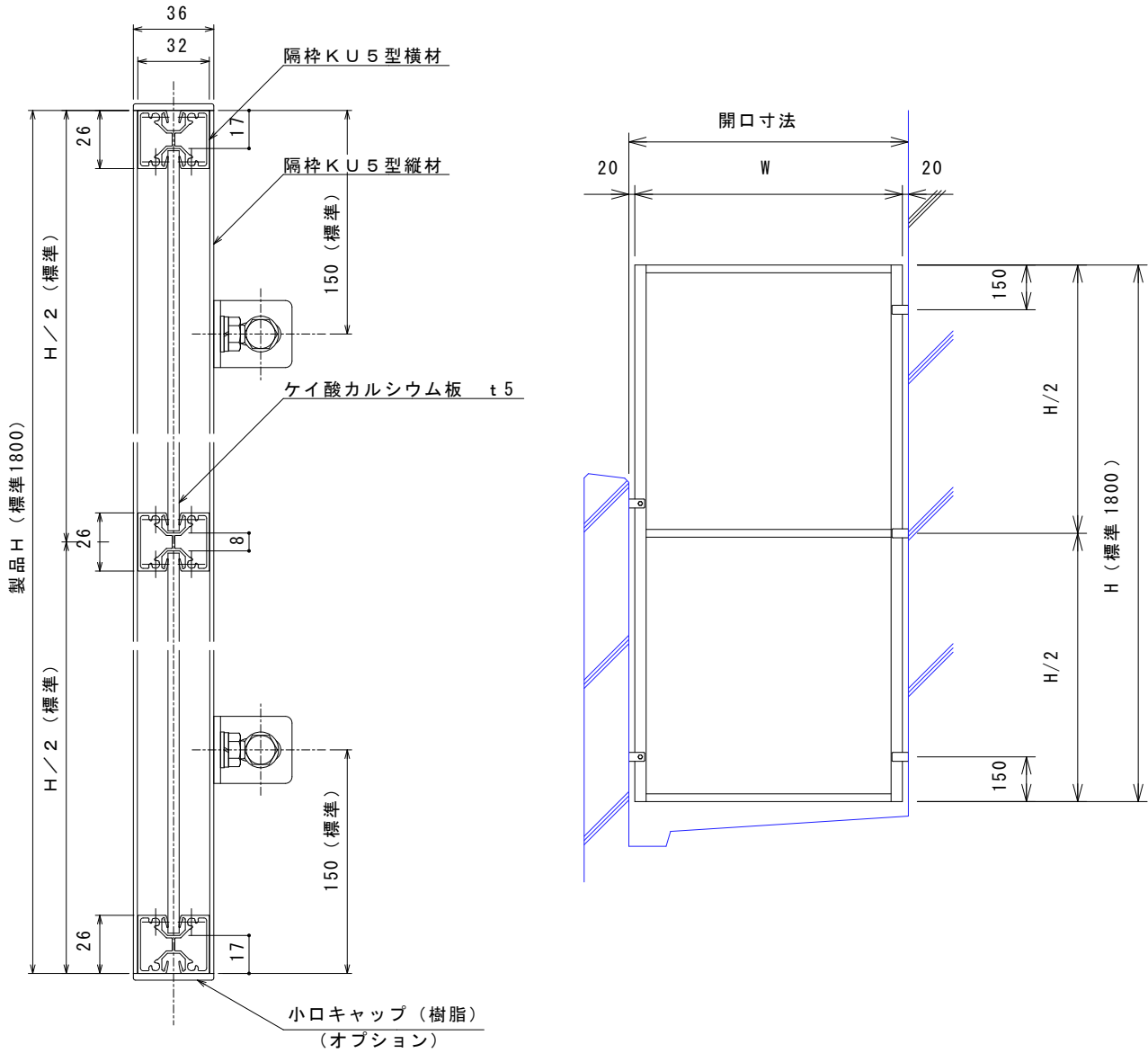
【 縦断面詳細図 】
